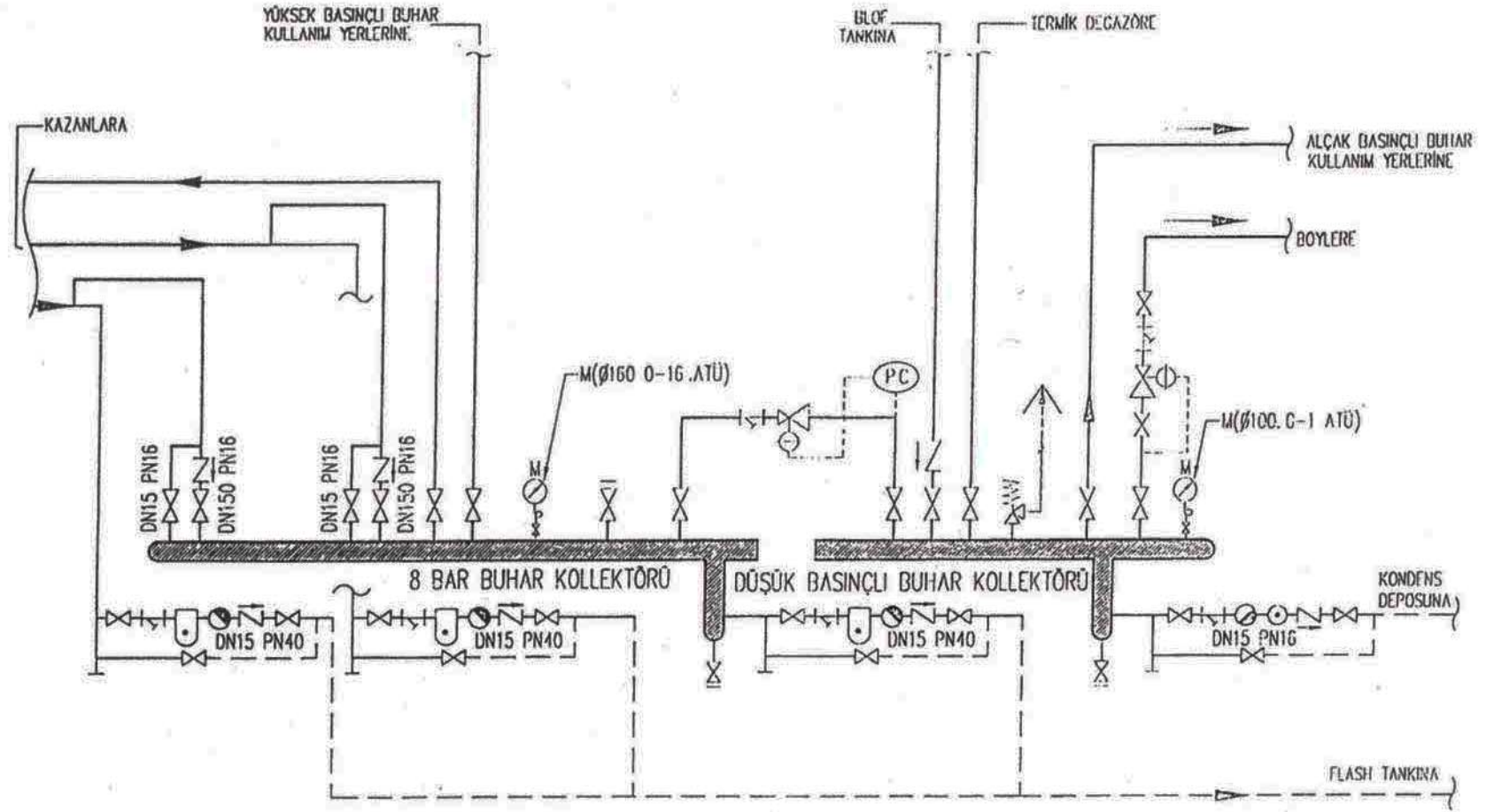
Yüksek ve Alçak Basıncı Buhar Kollektörleri
