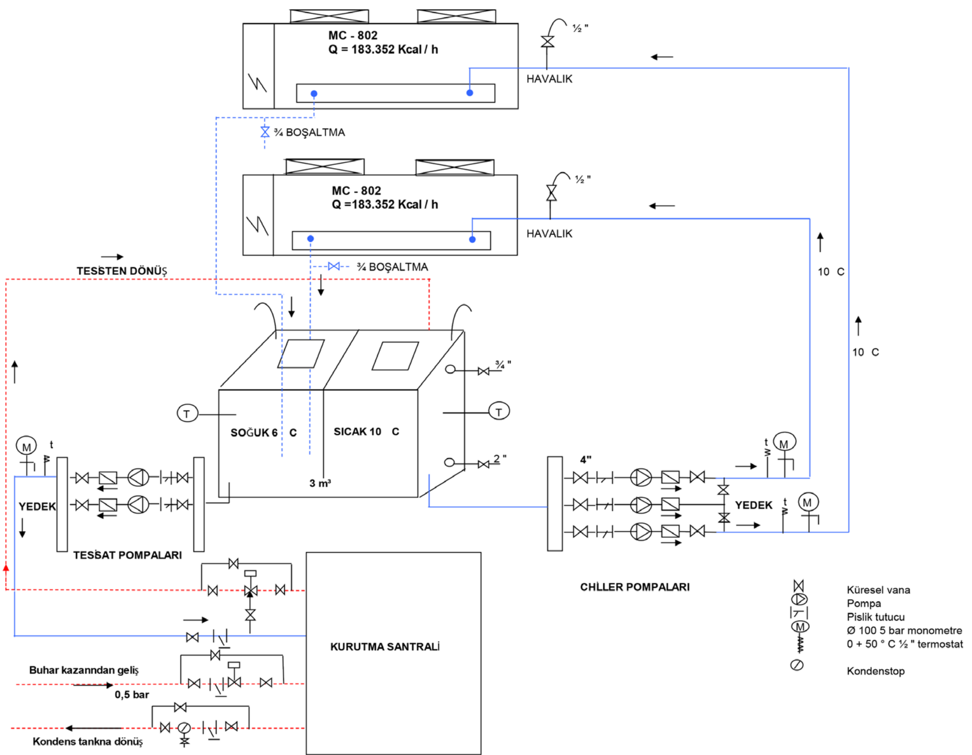
AKIŞ TP, REGÜLASYON TANKLI, PROSES SANTRALLİ CHLLER, CHLLER POMPALARI, TESSAT POMPALARI, BAĞLANTI PRENSP ŞEMASI
