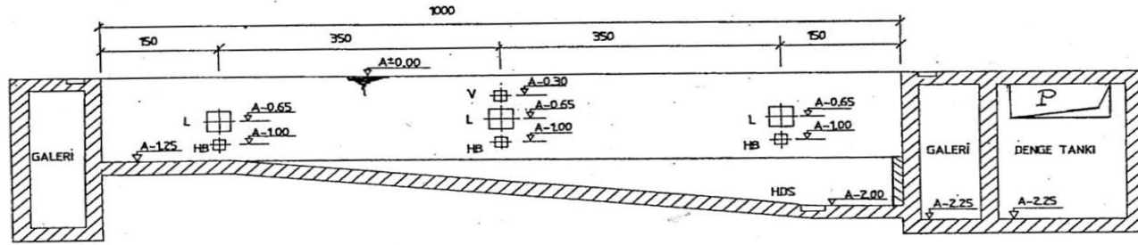
A-A KESİTİ
